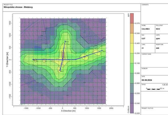
Рис. 8. Модель розповсюдження NO 2 перехрестя просп. Металургів і Нікопольського шосе
