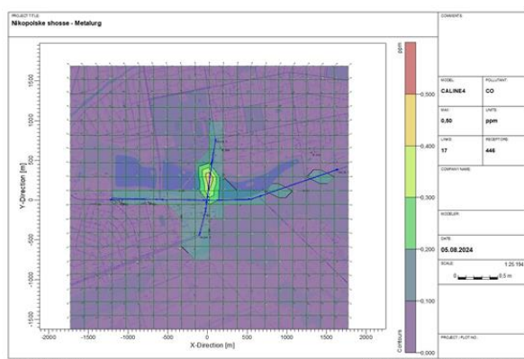
Рис. 7. Модель розповсюдження CO перехрестя пр. Металургів і Нікопольського шосе
