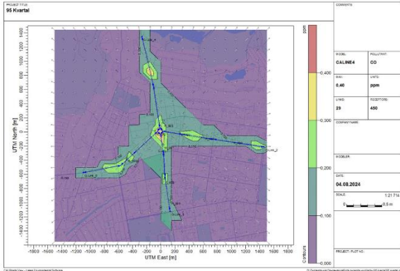
Рис. 3. Модель розповсюдження CO 95 квартал
