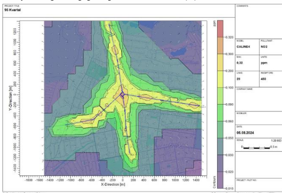
Рис. 4. Модель розповсюдження NO 2 95 квартал
