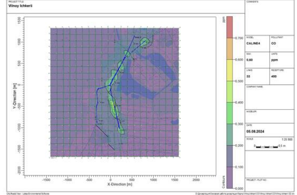
Рис. 5. Модель розповсюдження CO вул. Вільної Ічкерії
